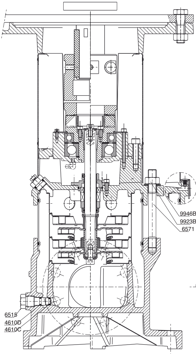
MULTI-V 36C DN65 - PN25
